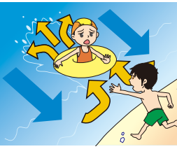
離岸流
