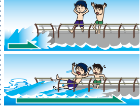
潮汐
